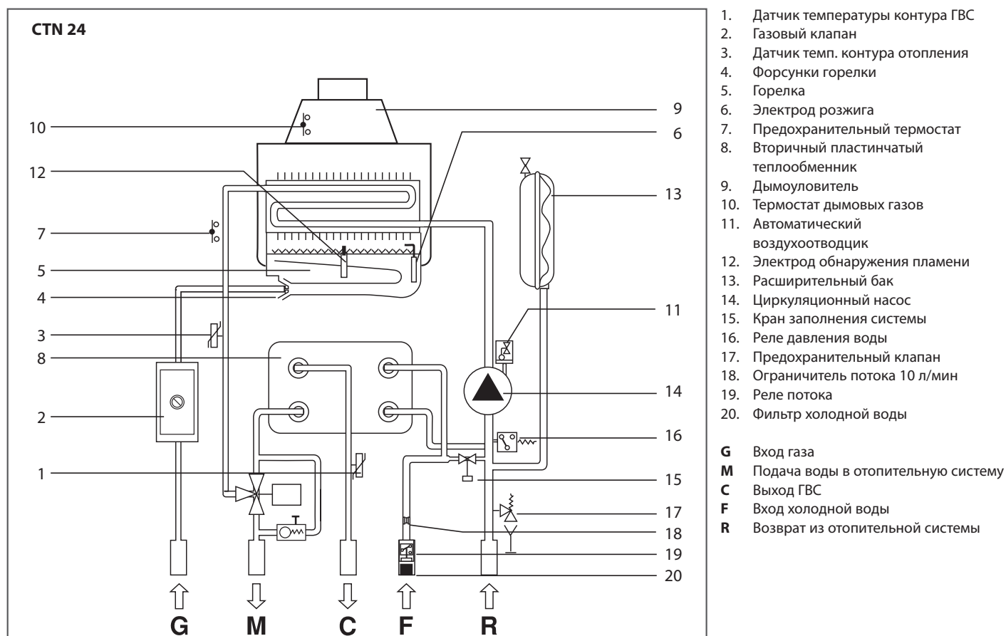
рис. 6 - Гидравлическая схема мод. CTN 24
